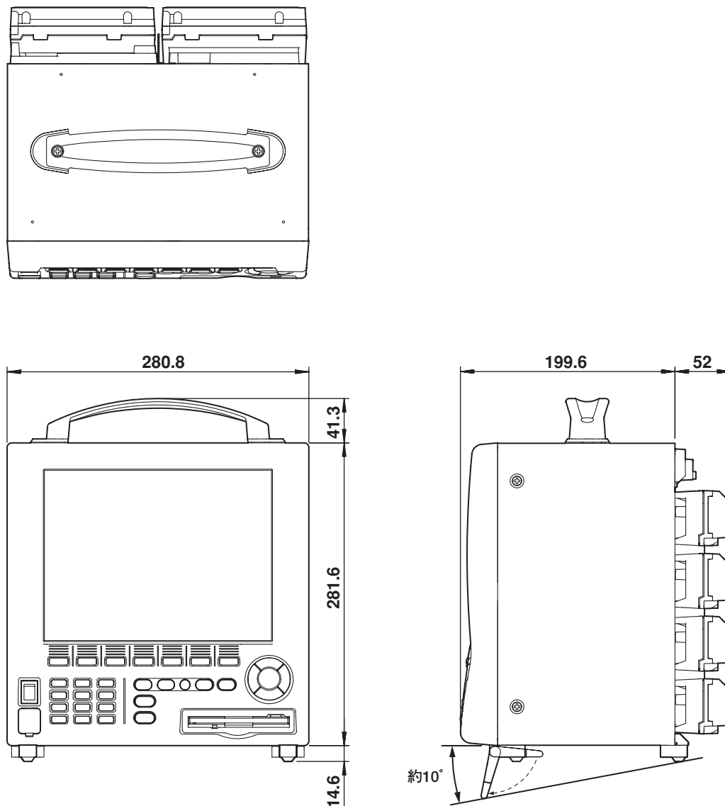
外形図
