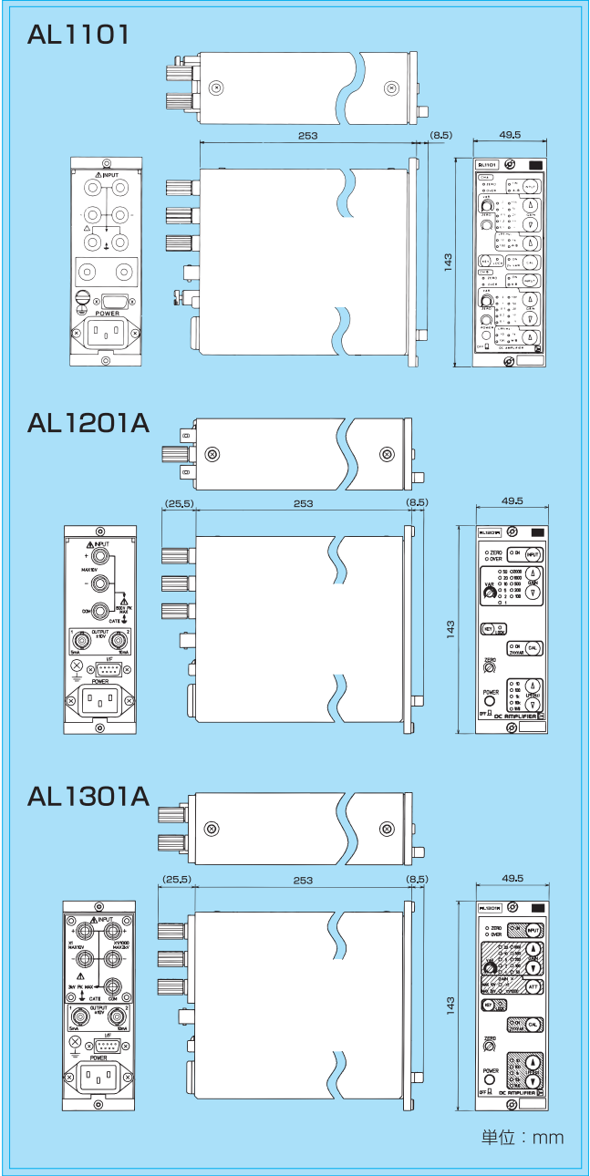
ALシリーズ外形寸法図
