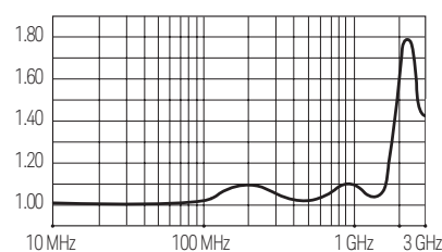
VSWR
