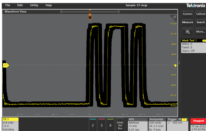
高品質なリファレンス信号に基づくリミット・マスク・テスト
