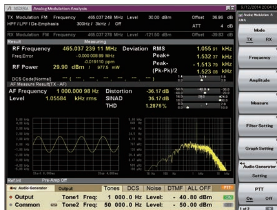
AF信号出力(下側)とFM変調信号測定(上側)の測定例
