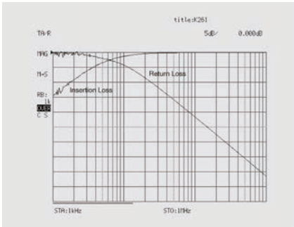
低い周波数挿入損失とリターンロス (代表値) K261、1 kHzから1 MHzの範囲で測定 K261 精密DCブロック リターンロス
