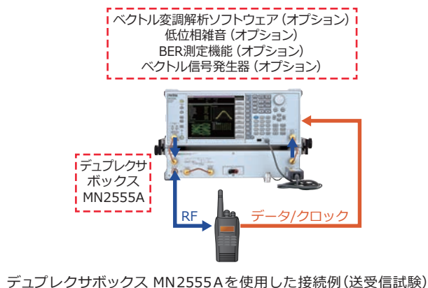
デュプレキサボックス MN2555Aを使用した接続例(送受信試験)
