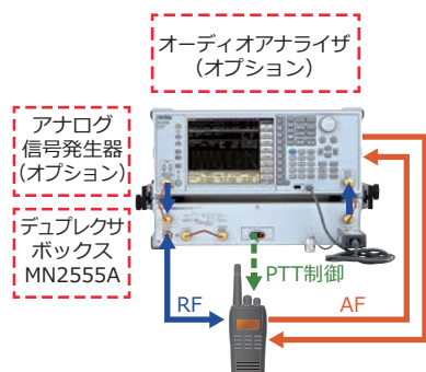
デュプレクサボックス MN2555Aを使用した接続例(送受信試験)
