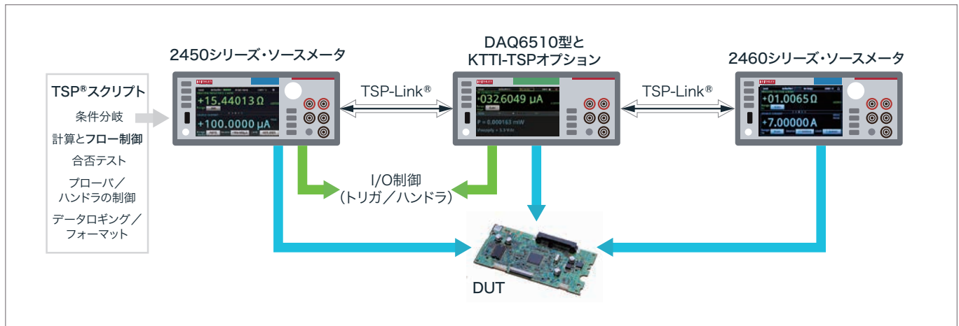
TSP-Linkを使用した、TSPシステムによる機器間の通信
