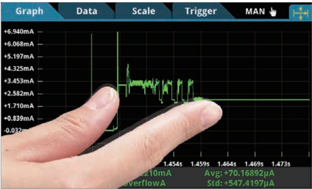
ピンチ／ズームによる簡単な操作で詳細な波形解析が可能
