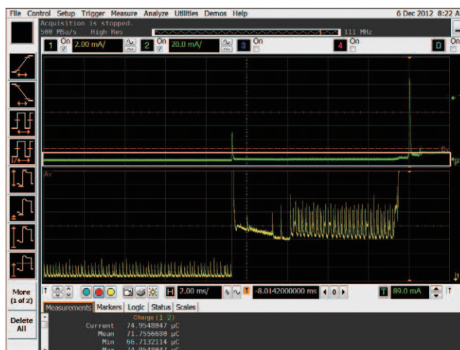
図5. InfiniiumオシロスコープとN2820A電流プローブを組み合わせれば、波形の下面積を計算して、正確な消費電流を求めることができます。
