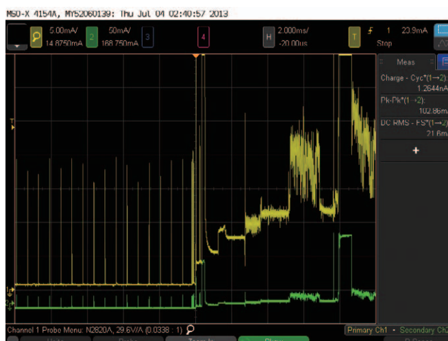
図6. InfiniVision 3000 X/4000 XシリーズオシロスコープでN2820Aを使用すると低利得ビューと高利得ビュー(N2821Aの場合はどちらか一方のビュー)を同時に表示でき、よりダイナミック・レンジの広い電流測定が行えます。
