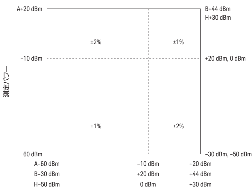
図2. EPMシリーズパワー・メータの25℃ ± 10℃での相対モードでのパワー測定リニアリティ(代表値)
