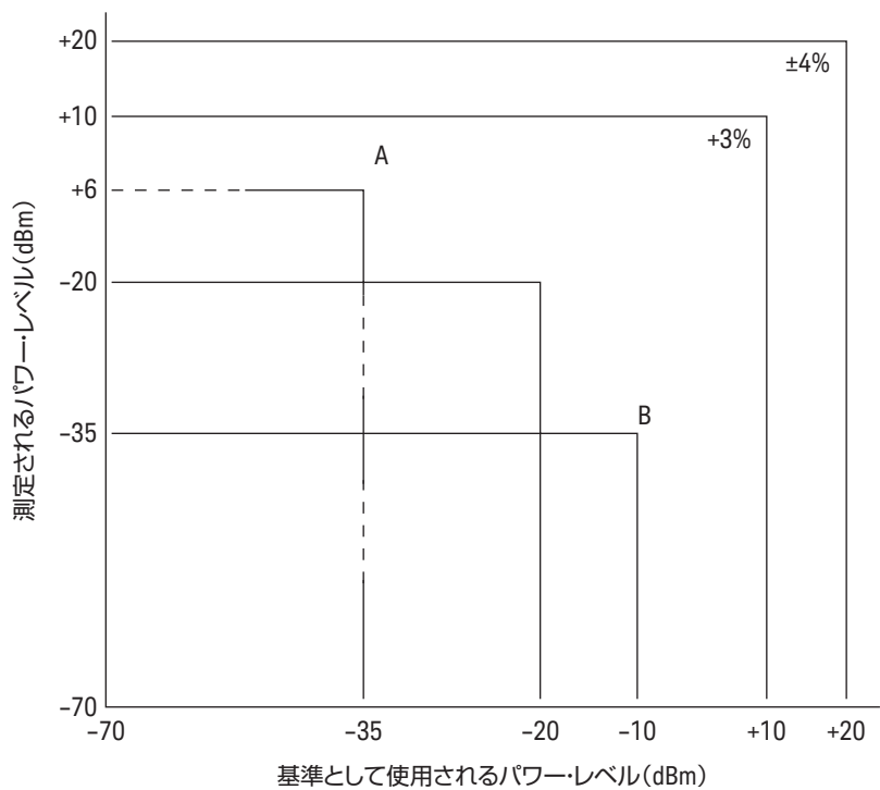
図1. EPMシリーズパワー・メータ/EシリーズCWパワー・センサの相対モードでのパワー測定リニアリティ (25℃±5℃、代表値)
