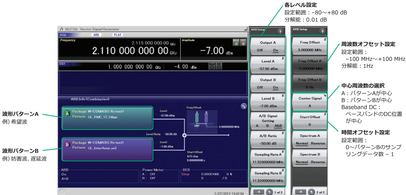
ベースバンド信号加算の一例
