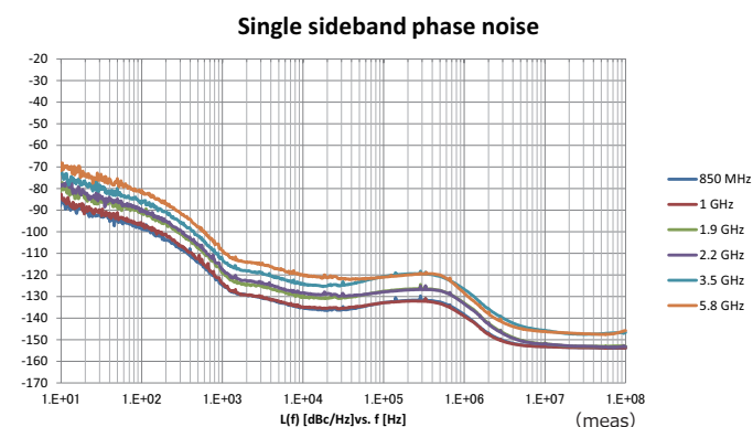
SSB位相雑音の一例 (Phase Noise Optimization <200 kHz、CW、Optimize S/N Off、 オプション002搭載時)
