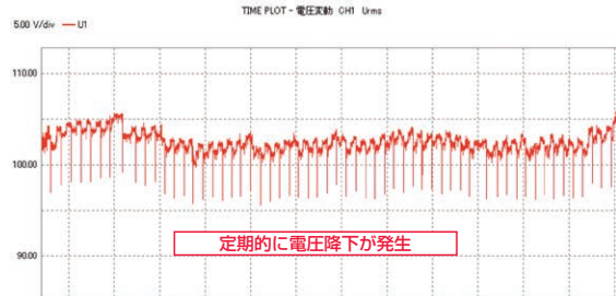
電圧変動グラフ
