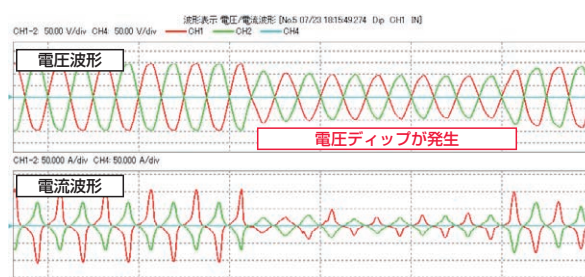
電圧ディップ発生時の電圧波形と電流波形
