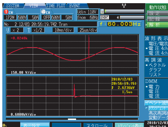
トランジェントオーバ電圧 (インパルス)
