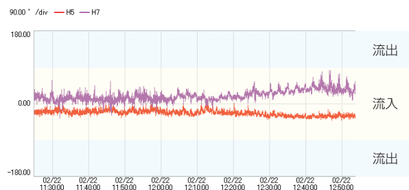
流入 / 流出判定の例（5次、7次高調波が流入）
