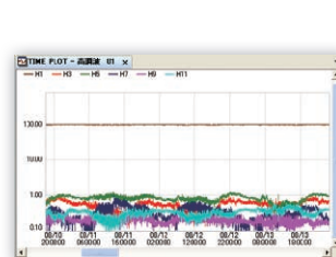
高調波時系列画面
